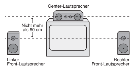
A) Aufbau des Center- und der Front-Lautsprecher in der Nähe eines Fernsehers oder Rückwandprojektors.
