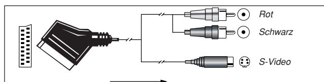
Abbildung 4: SCART/S-Video Adapter für Wiedergabe; Signalfluss: SCART → Cinch und Mini-DIN
